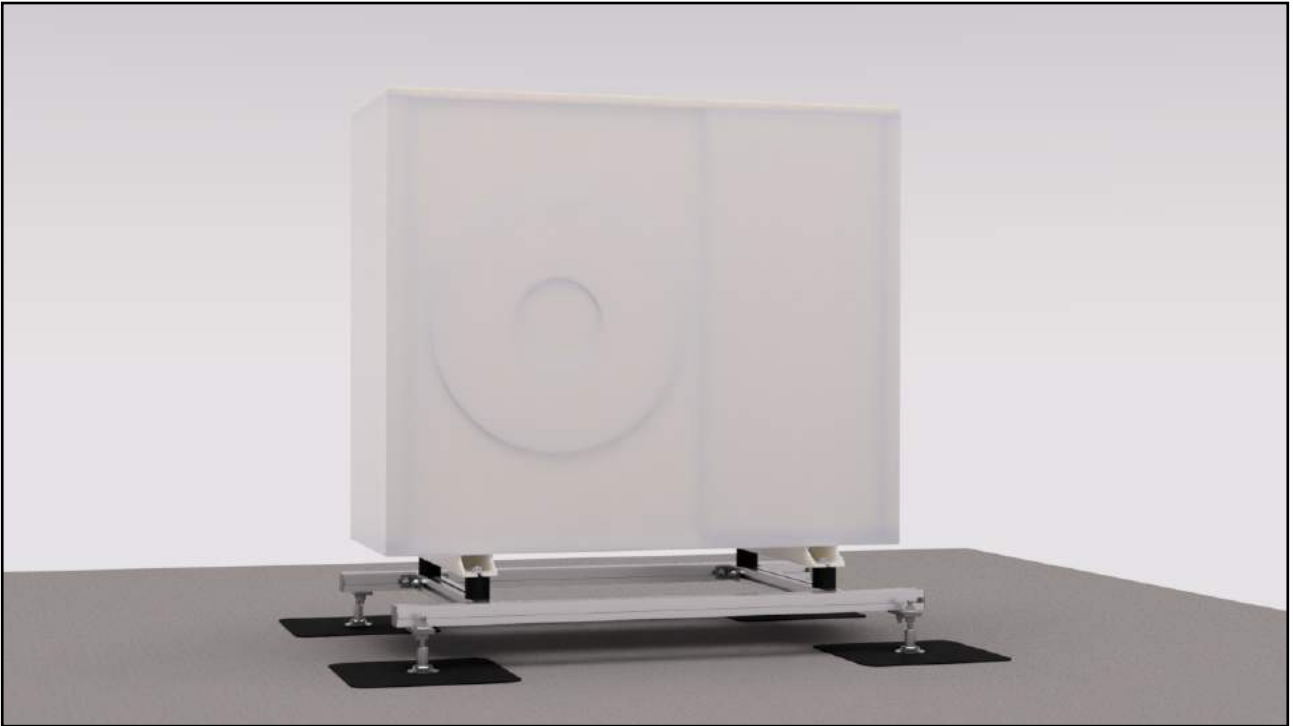
ROOFSOLUTIONS - Montagerahmen für Wärmepumpen / mounting frame for heat pumps Montageanleitung / Installation manual
